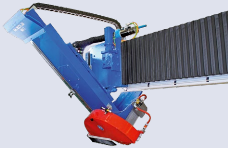
Schwenksupport 0 - 45° (Gehrungsschnitt) (optional)
